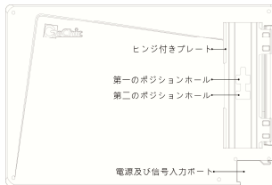
図：0n-Lapの背面
